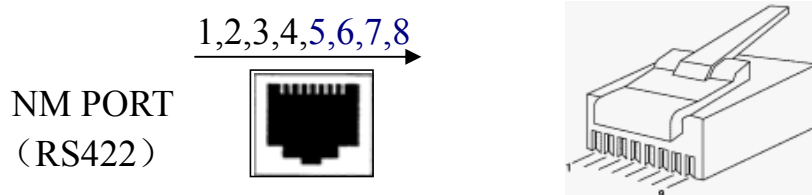
RJ45 插座管脚排列图
